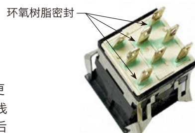
变更前端子底部的环氧树脂密封示例
