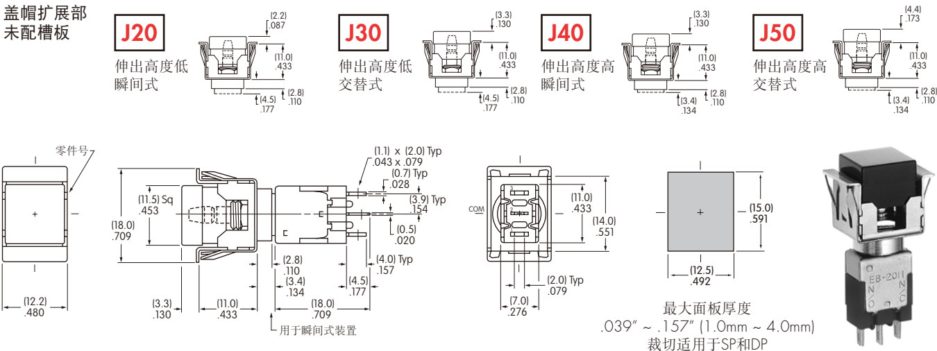
伸出高度高 单极 EB2011-A-J40
