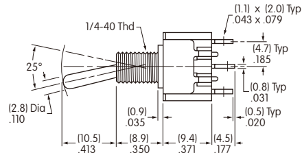
M2011型没有端子1。
