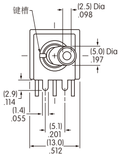
单色LED开关没有端子5。
